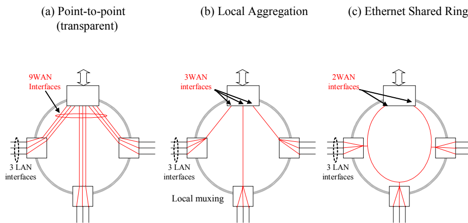
Рис. 1.3. Три режима передачи трафика Ethernet мультимплексорами FG-FOM2,5G.L2.
