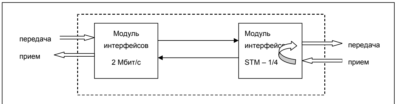
Рис. 15. Тестирование волоконно-оптической линии и интерфейсного модуля STM-1/4 удаленного мультиплексора
