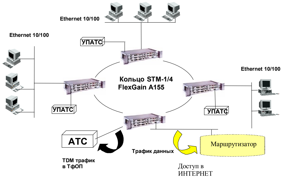
Рис. 5. Объединение локальных корпоративных сетей
