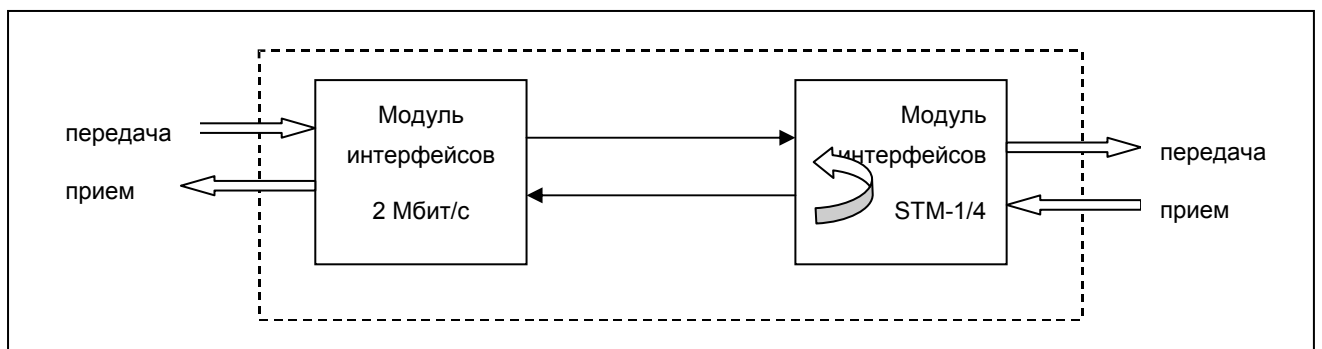
Рис. 16. Тестирование интерфейсного модуля STM-1/4 ближнего мультиплексора
