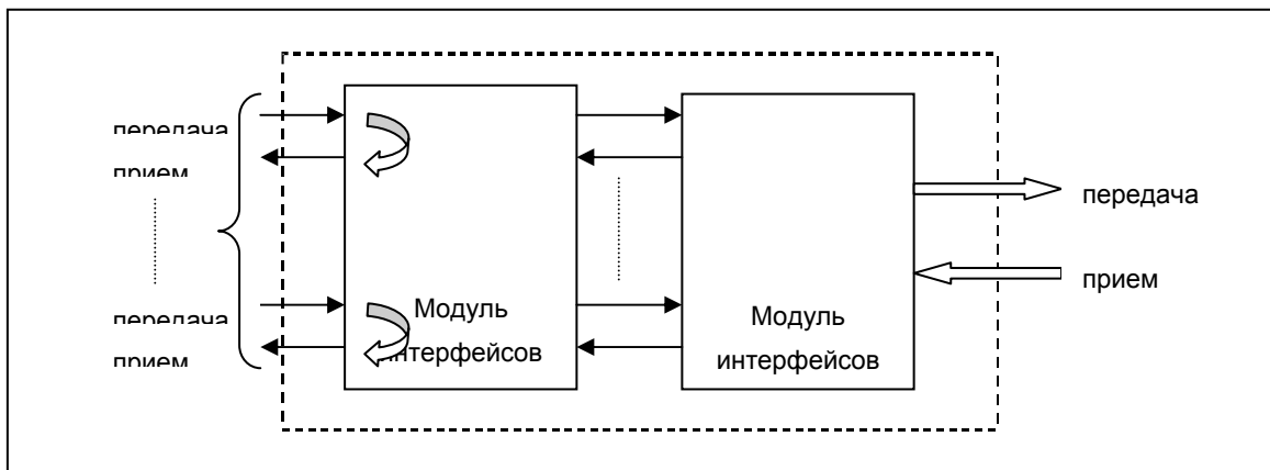
Рис. 17. Тестирование интерфейсных модулей компонентных потоков 2/34/45 Мбит/с ближнего мультиплексора.
