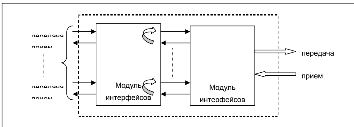
Рис. 18. Тестирование интерфейсных модулей компонентных потоков 2/34/45 Мбит/с удаленного мультиплексора
