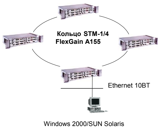
Рис. 14. Организация доступа для централизованного управления SDH-сетью
